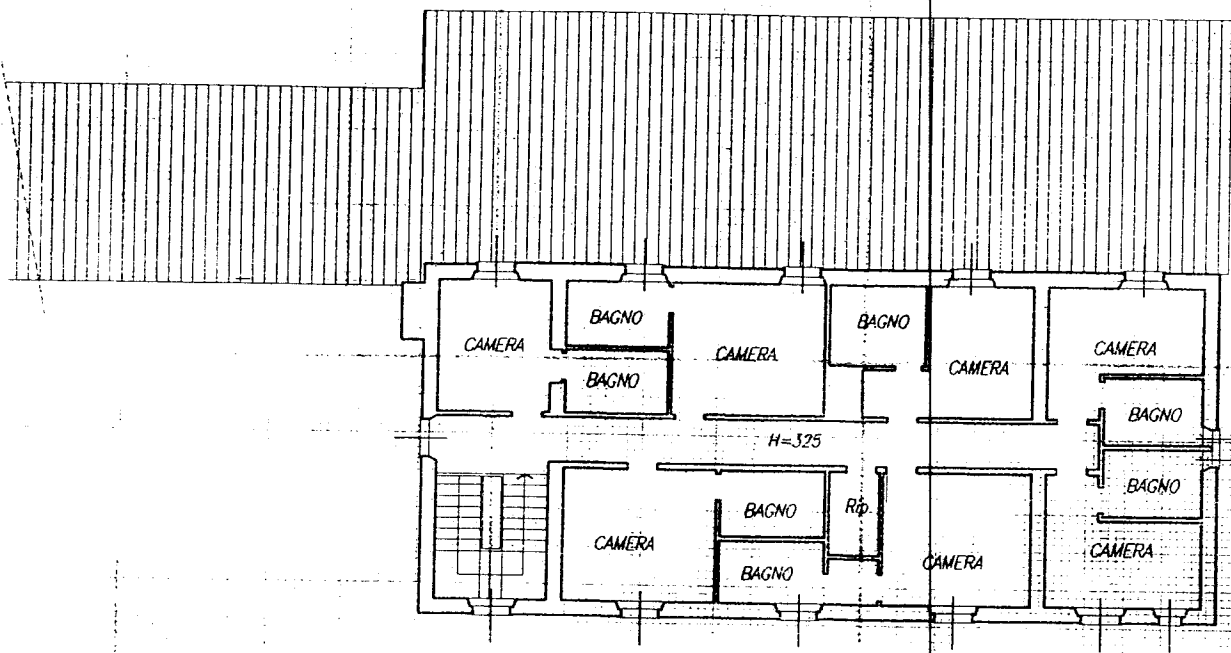
PIANTA PIANO PRIMO CORPO A
